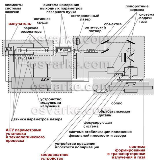
Рис. 1 Принципиальная схема устройства лазерно-гравировальной машины
