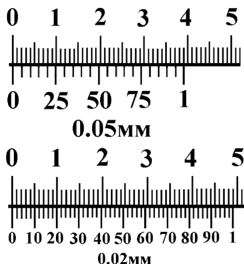
Рис. 1- Измерительная шкала нониуса (нулевое положение)
