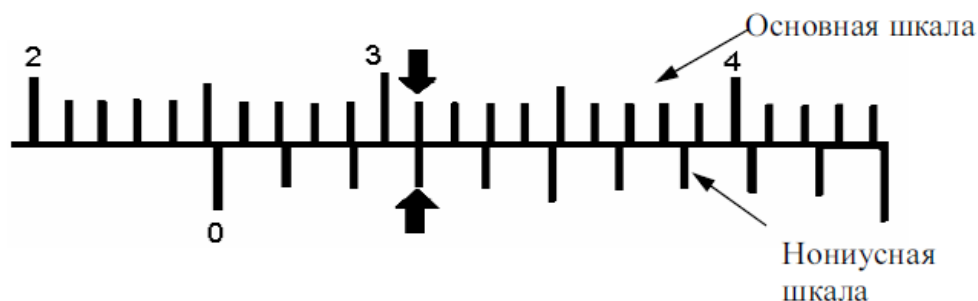
Рис. 2 - Показание штангенциркуля (25,3 мм) с ценой деления по нониусной шкале 0,1 мм (по основной шкале – 25,0 мм, по нониусной шкале – 0,3 мм)
