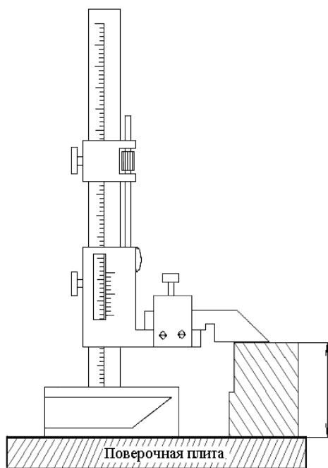
Рис. 11 – Прием измерения
