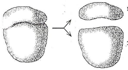
Рис. 7. Строение рибосомы.
