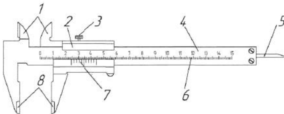
Рис. 3 - Штангенциркуль ШЦ I двусторонний с глубиномером
