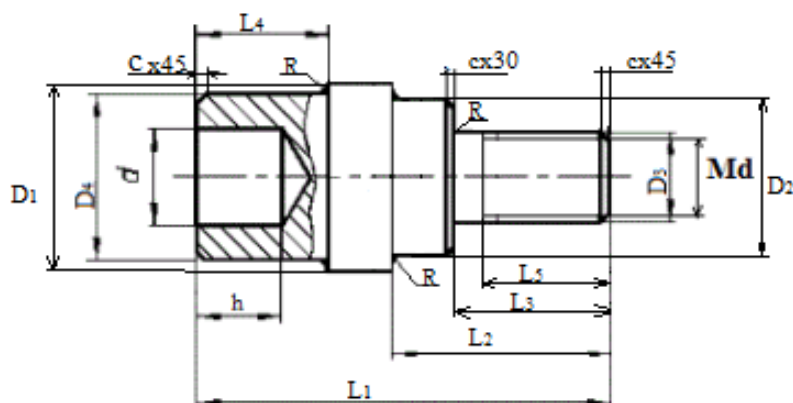
Рис.13 – Эскиз детали
