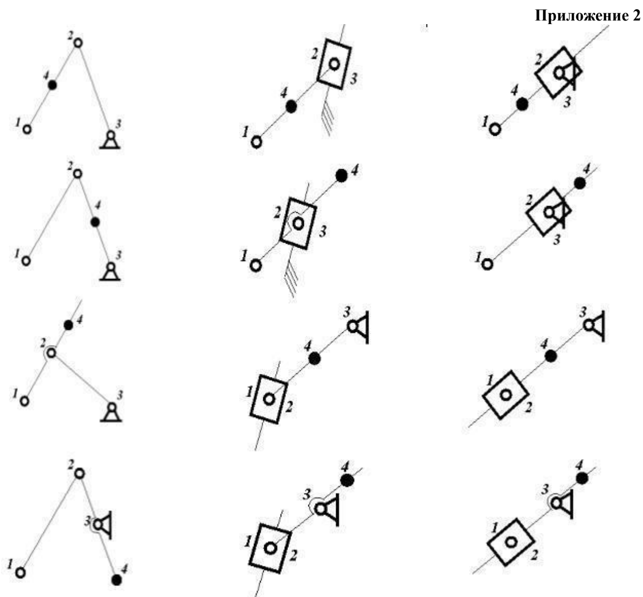
Рис.1. Синтез кинематической схемы механизма
