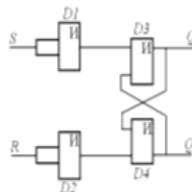
Рис.6. Логическая схема триггера [15]
