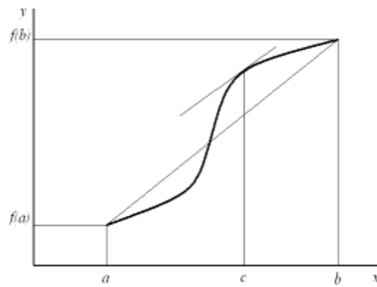
Рис.3. Геометрический смысл теоремы Лагранжа [5]
