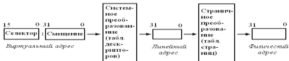
Рис.7. Схема преобразования виртуального адреса в физический [16]
