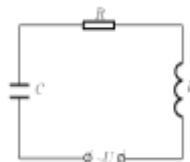
Рис.5. Схема колебательного контура [14]
