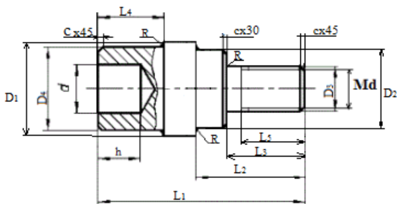
Рис.13 – Эскиз детали
