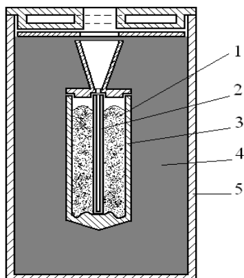
Рис.1. Устройство светового эталона фотометрической единицы [11]:
