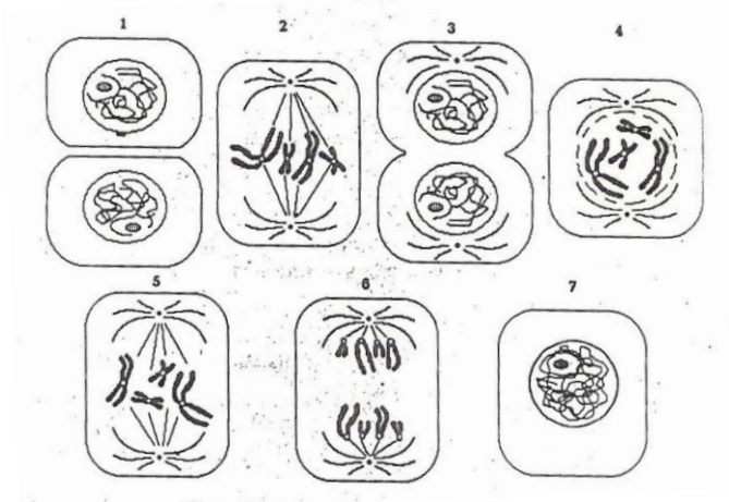
Рис. 13. Схема фаз митоза.
