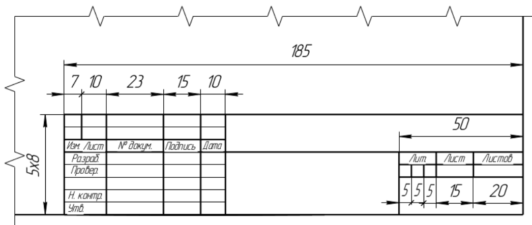
Рисунок 13 Основная надпись для первого листа текстовой документации (форма 2)
