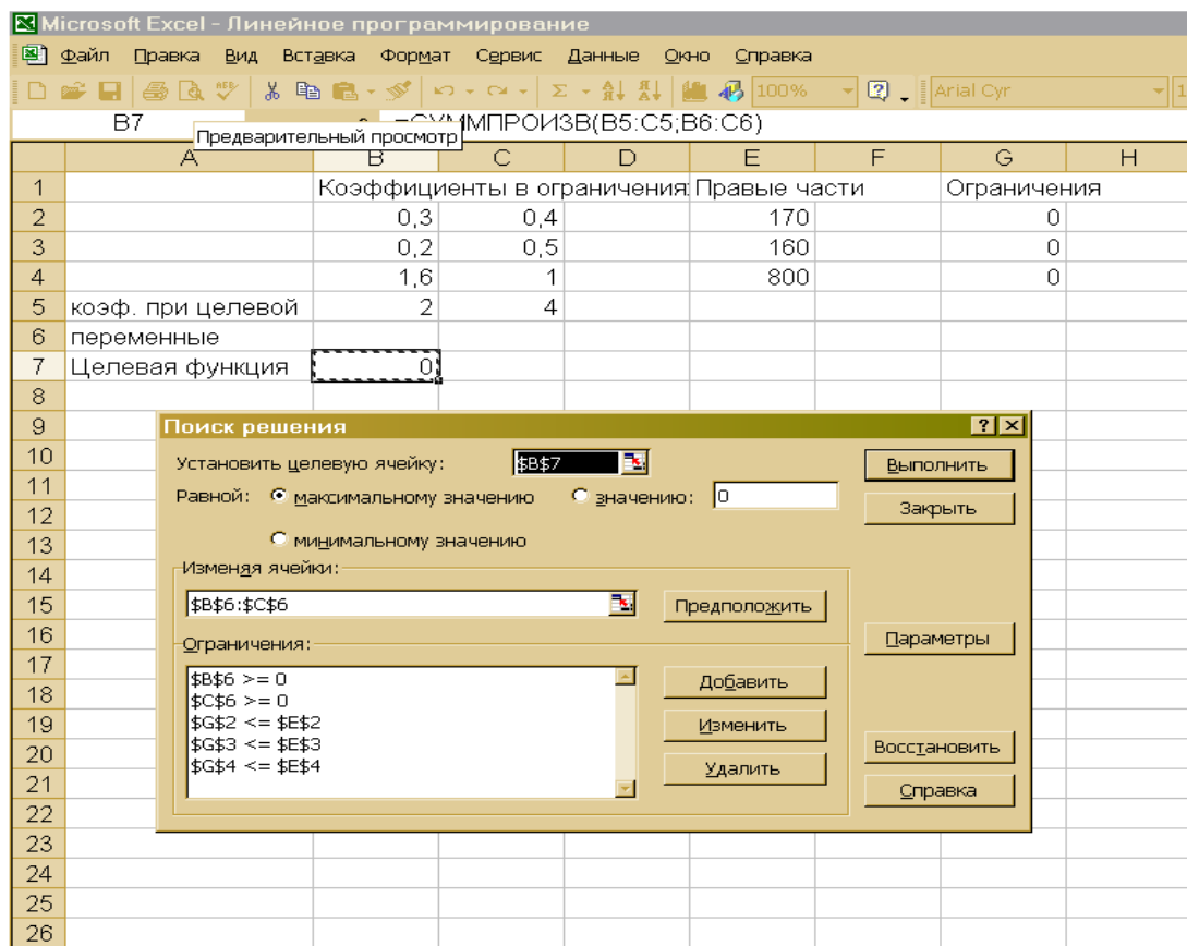
Рис. 2. Фрагмент Листа Excel на экране с диалоговым окном Поиск решения
