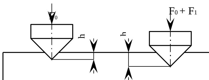
Рис. 2. Схема определения твердости материалов методом Роквелла Глубина вдавливания индентора автоматически измеряется прибором
