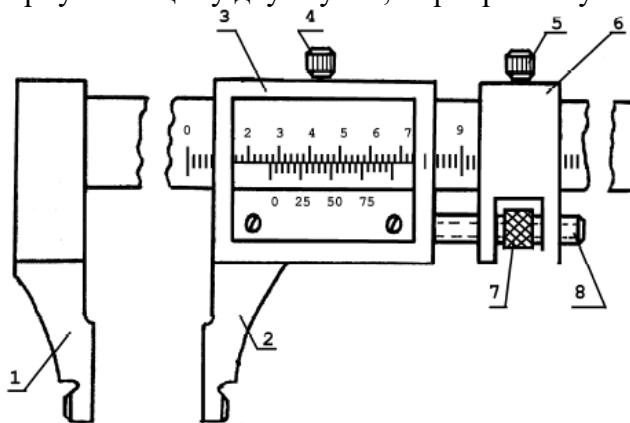
Внутренние плоскости губок 1 и 2 служат для наружных измерений, наружные цилиндрические поверхности – для внутренних измерений. К отсчету по шкале с нониусом следует прибавлять суммарную толщину двух губок, маркированную на них.
